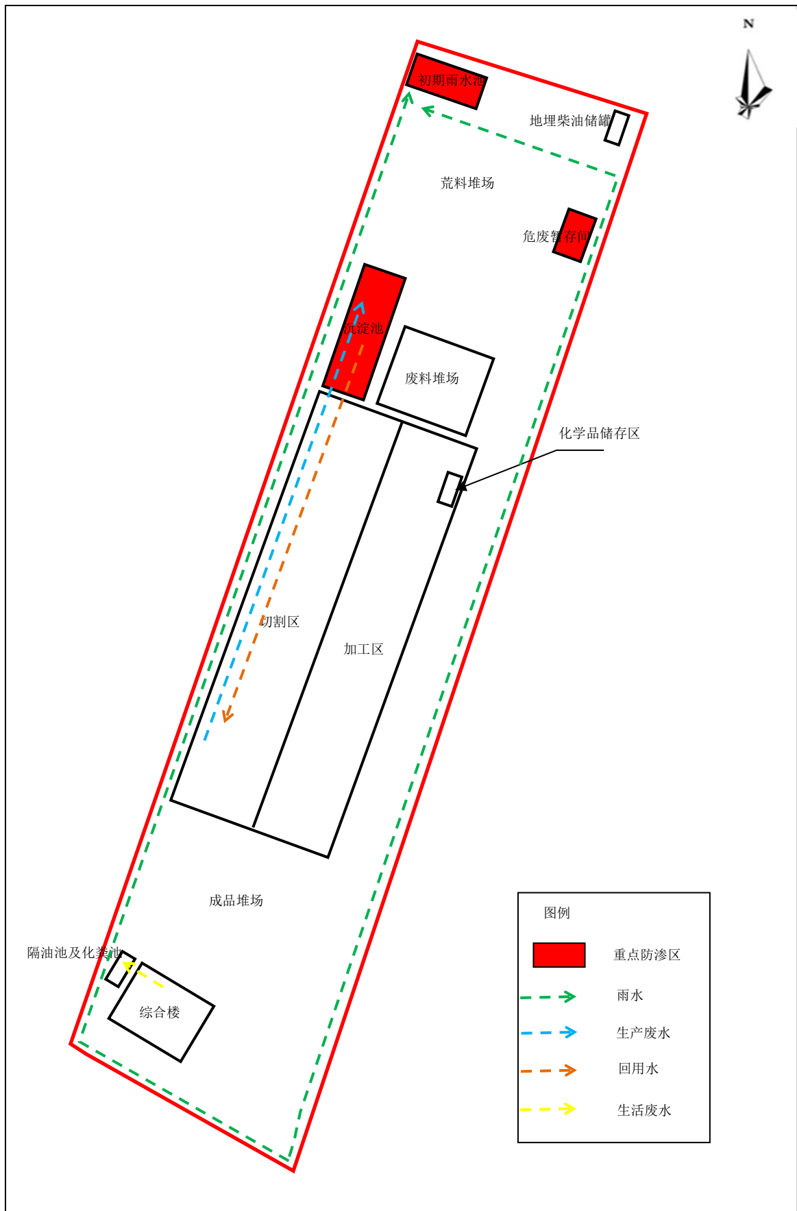
附图3 项目平面布置图及雨污管网图
