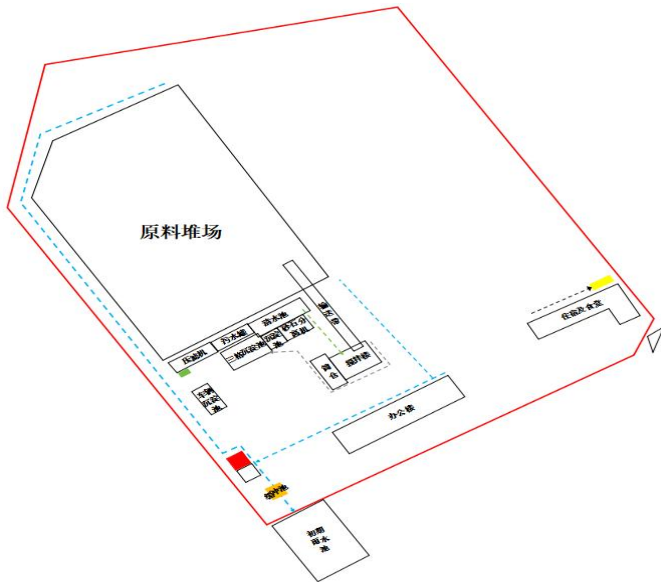
附图 3 项目总平面布置图及雨污管网图
