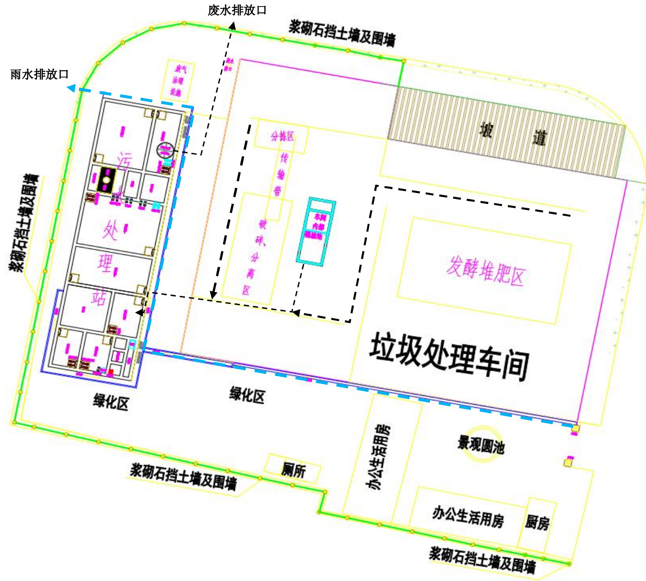
附图 4 项目雨污管网图
