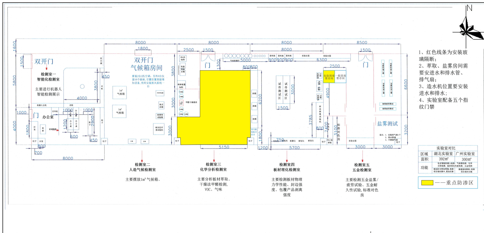
附图 4 实验室平面布置图及分区防渗图
